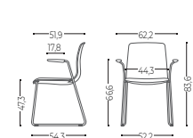
Cantilever with simple arm Patin metálico con brazo simple
