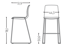
Cantilever stool without arms Taburete patin metálico sin brazos
